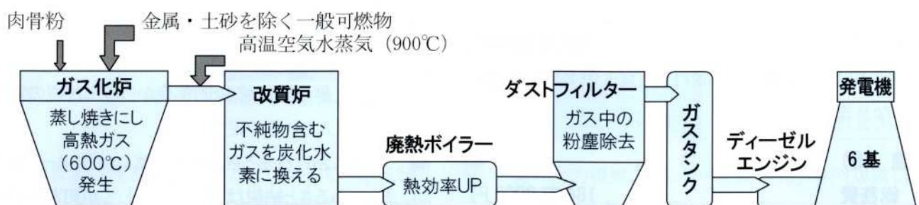
市来一般廃棄物利用エネルギーセンター設計略図
