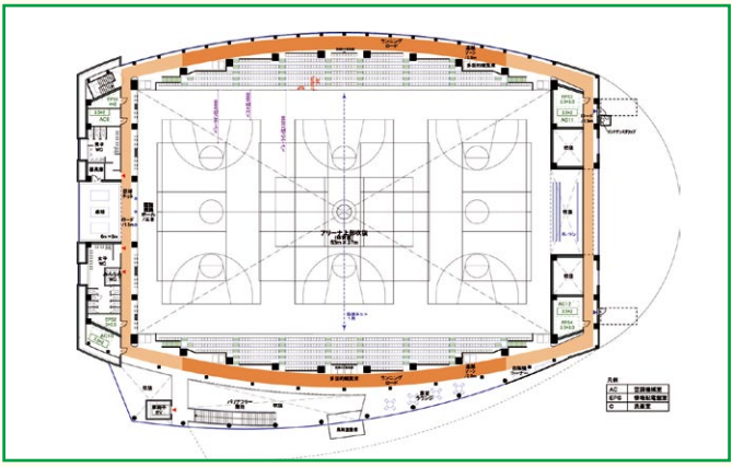
【完成平面図】 バレーボール 4面 バスケットボール 3面 バドミントン 14面・剣道 8面
