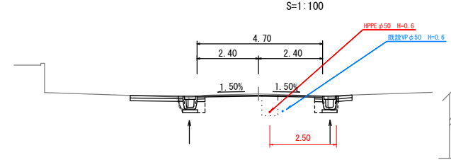
標準断面図
