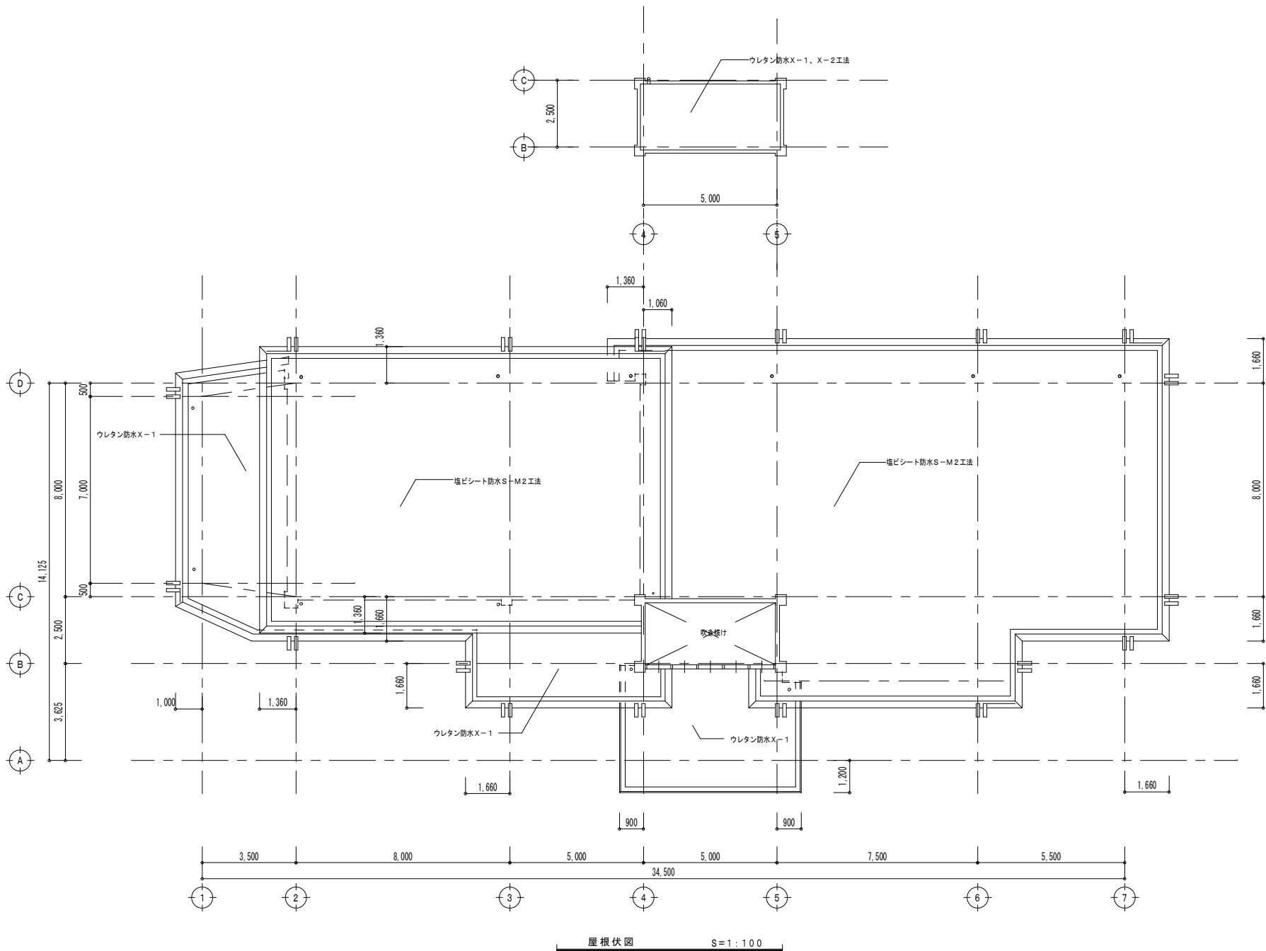
屋根伏図 S=1:100
