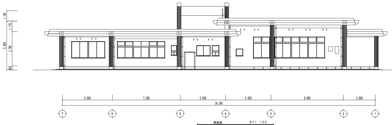
東面図 S=1:100
