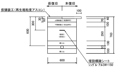
土工断面②(HPPEφ50) H=600 S=1:20
