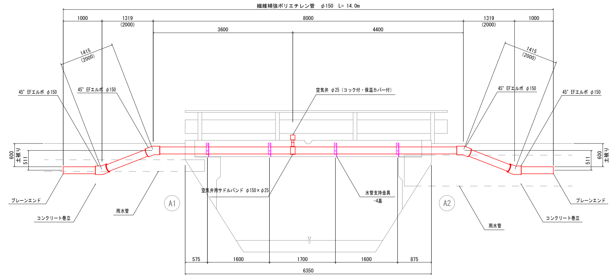
側面図 S=1:30
