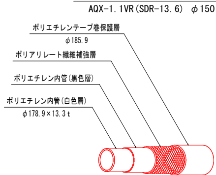
管断面詳細図 S=Free
