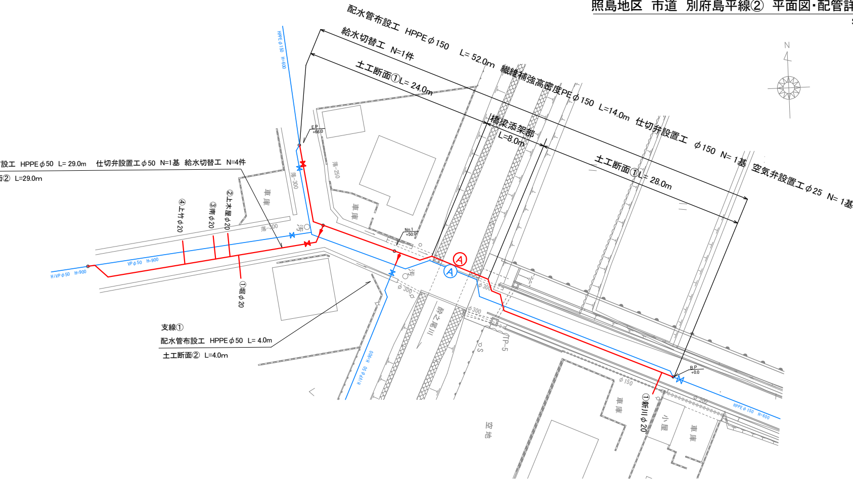
照島地区 市道 別府島平線② 平面図・配管詳細図
