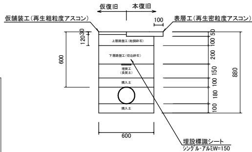
土工断面②(HPPE φ50)
