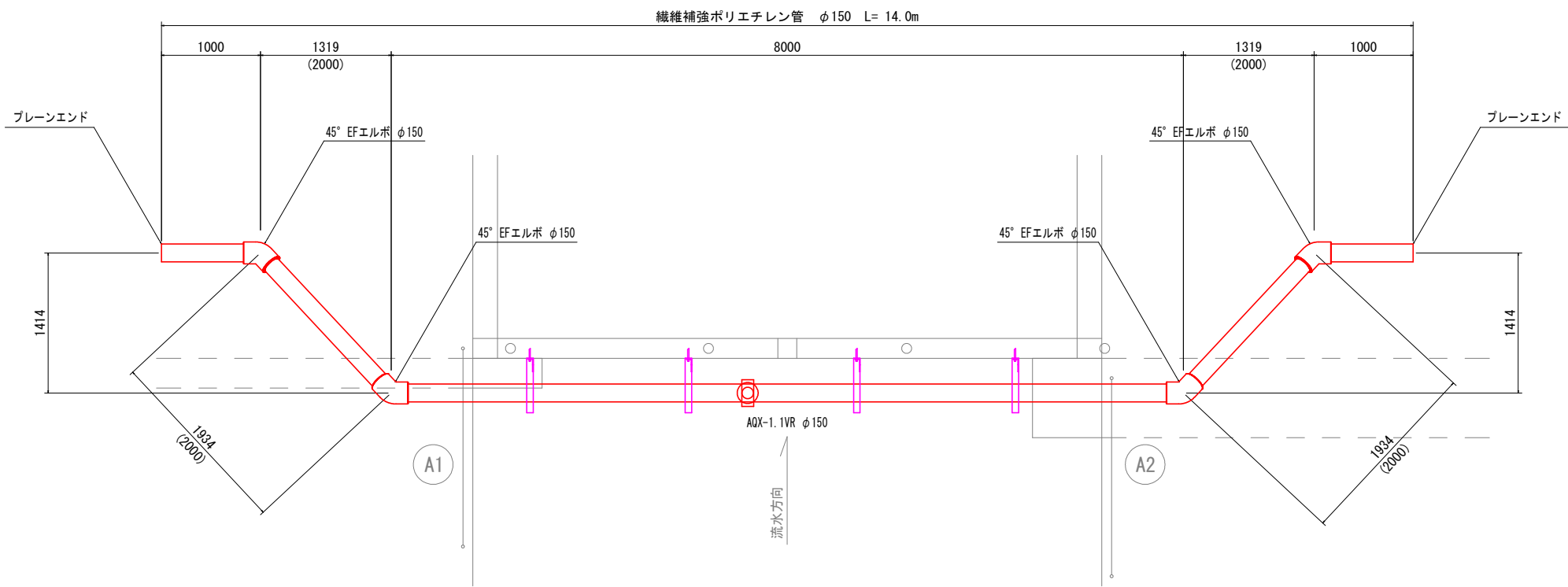
側面図 S=1:30
