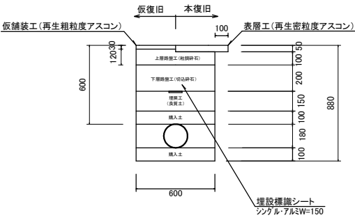
土工断面②(HPPEφ50) H=600 S=1:20
