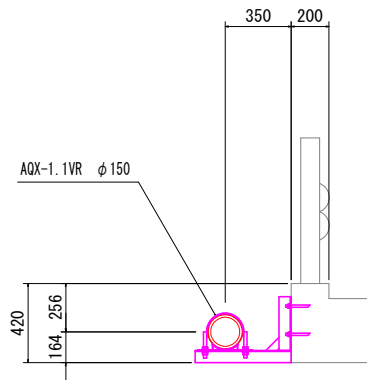
断面図 S=1:20
