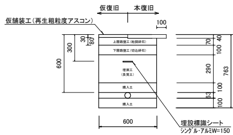
土工断面②(HPPE φ50)
