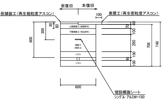
土工断面②(HiPV φ40) As舗装 H=600 S=1:20
