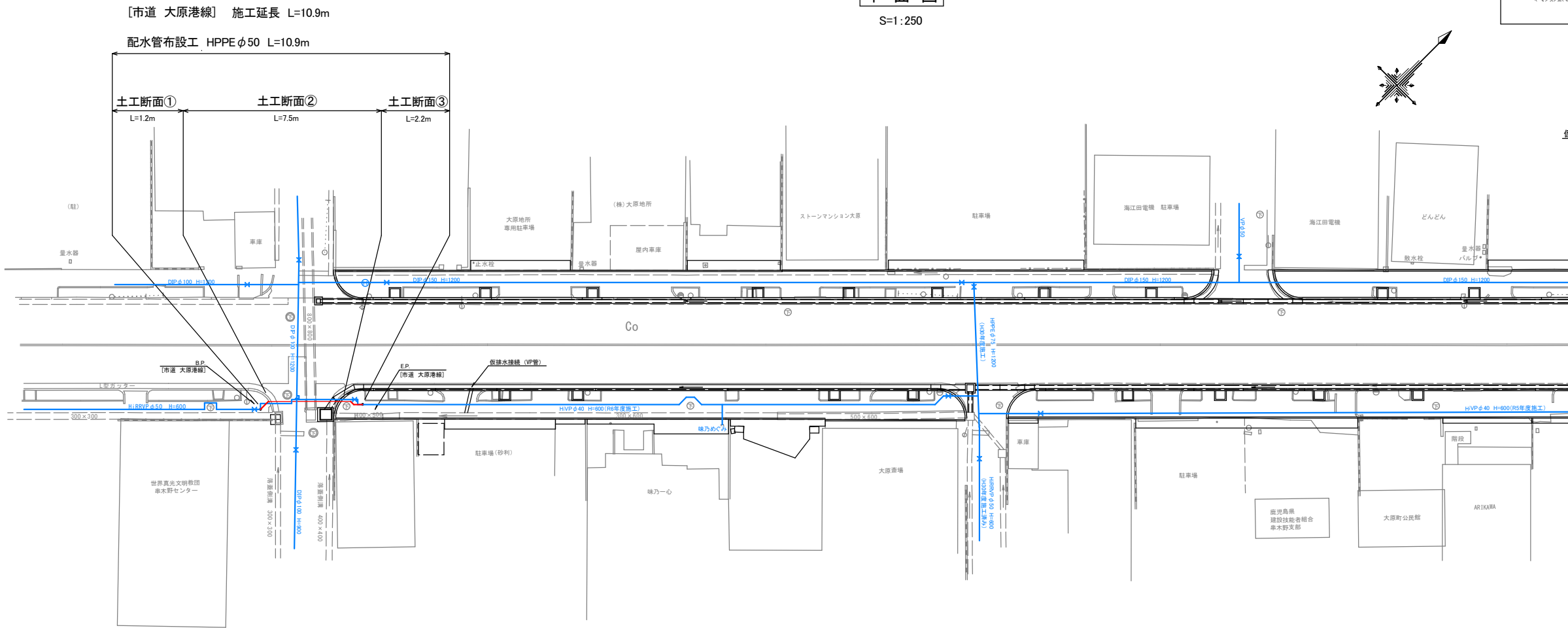
平面図
