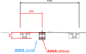
標準断面図 S=1:100 [市道 桜町大原線]
