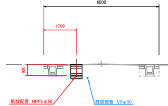
標準断面図 S=1:100 [市道 高見大原線-1]
