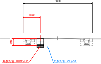
標準断面図 S=1:100 [市道 高見大原線-2]
