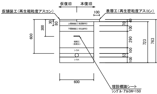
土工断面①(HPPE φ50) As舗装 H=600 S=1:20
