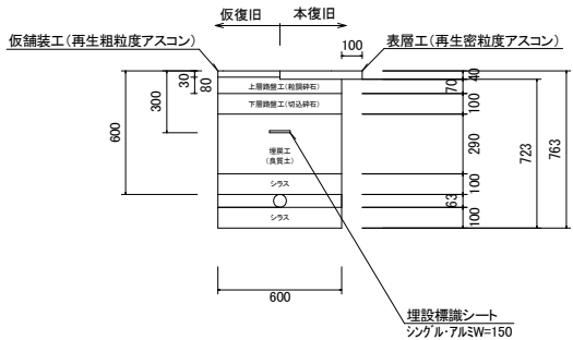
土工断面②(HPPEφ50) (市道)As舗装 H=600 S=1:20
