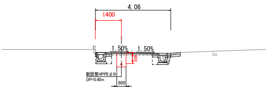
土工断面①(HPPE φ50)
