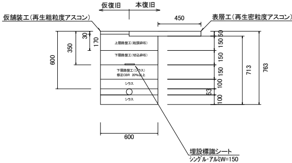
土工断面③(HPPEφ50) (県道)As舗装 H=600 S=1:20
