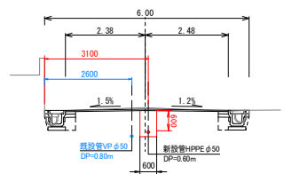
標準断面図
