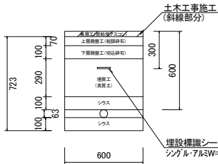
土工断面①(HPPEφ50) (市道)As舗装 H=600 S=1:20
