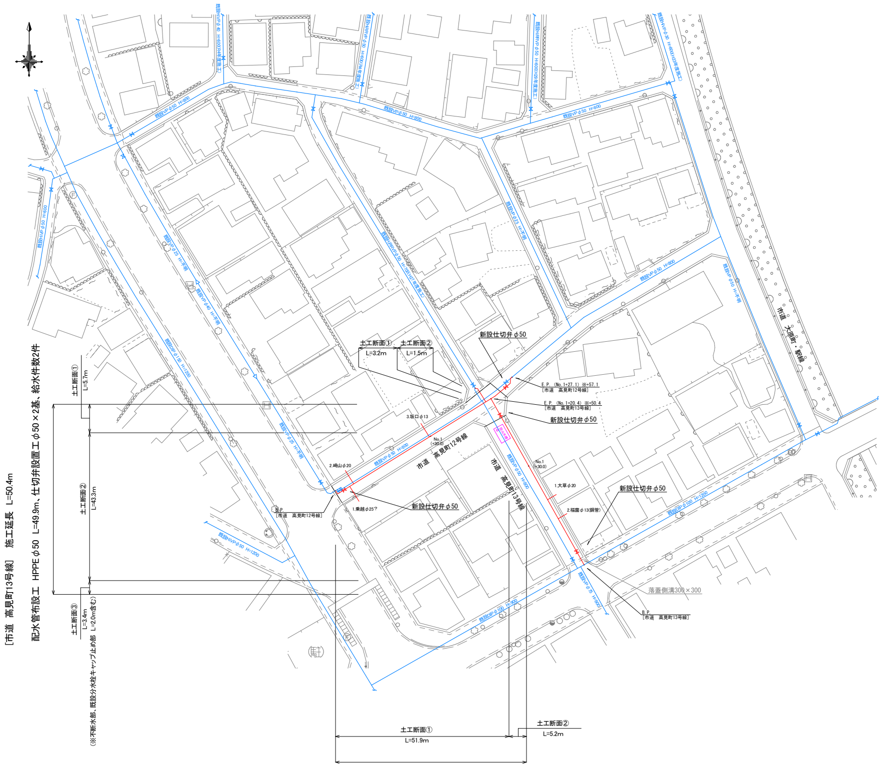
高見町 平面図 S=1:500 [市道 高見町12号線] [市道 高見町13号線]
