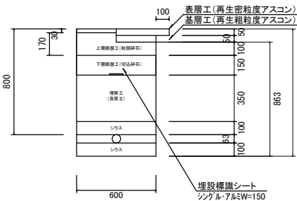
土工断面⑤(HPPEφ50) As舗装 H=800 S=1:20
