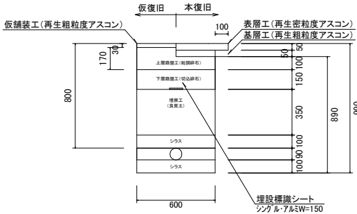
土工断面①(HPPEφ75) As舗装 H=800 S=1:20
