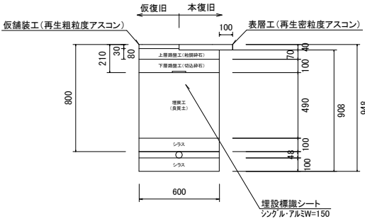
土工断面④(HiVPφ40) As舗装 H=800 S=1:20
