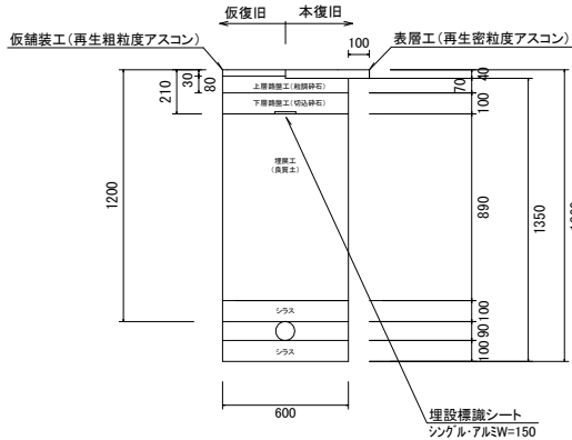
土工断面③(HPPEφ75) As舗装 H=1200 S=1:20
