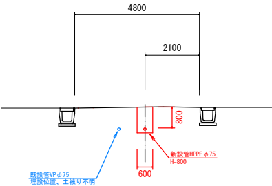
標準断面図(HPPEφ75)
