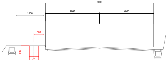
標準断面図 S=1:50 〔県道 戸崎湯之元停車場線〕
