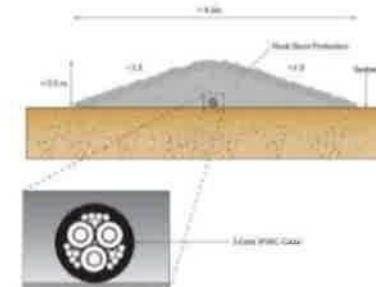
ケーブルを被覆した場合の断面(3)
