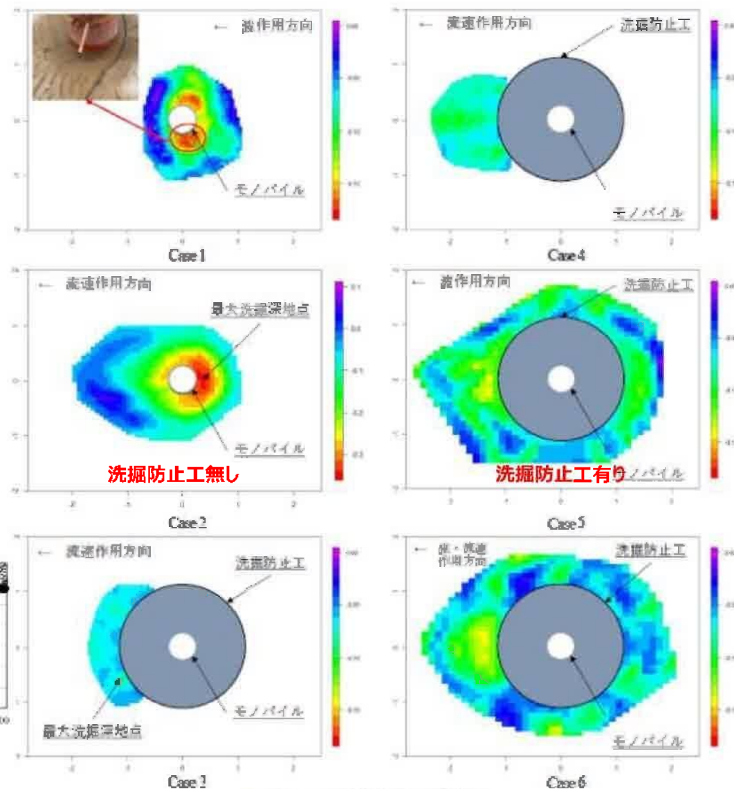
図6 各ケースの最終洗掘図 (単位: cm)
