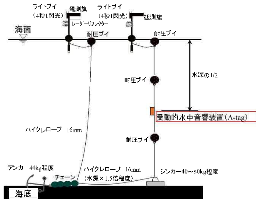
受動的な水中音響装置の設置イメージ
