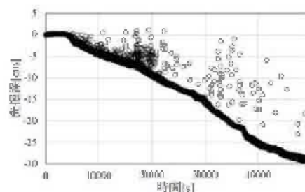
図4 Case2 (洗掘防止工無し)
