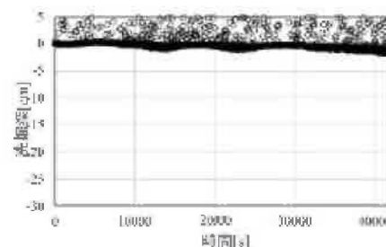
図5 Case3 (洗掘防止工あり)
