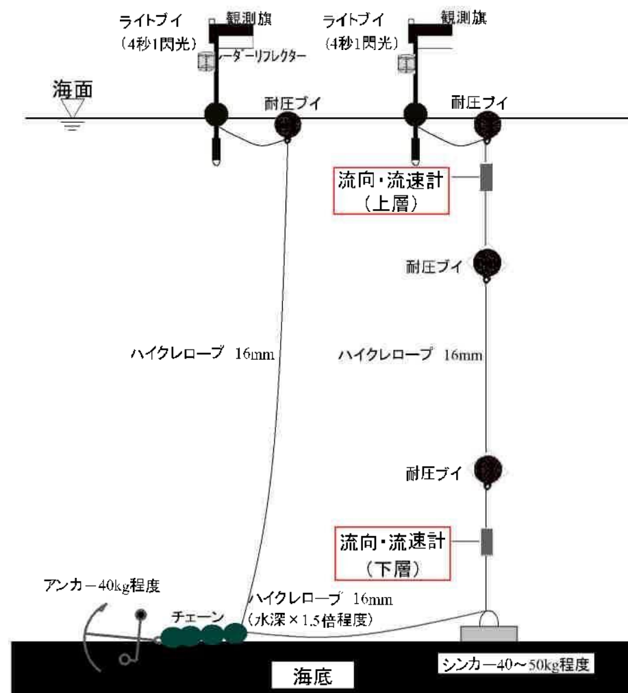
流向・流速計設置イメージ
