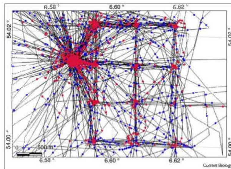
図 ドイツ国のAlpha Ventus洋上風力発電所におけるゼニガタアザラシの行動
