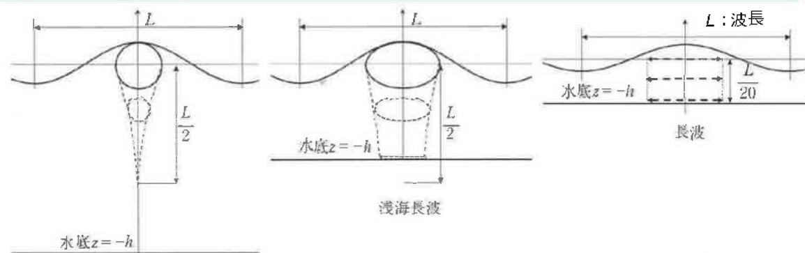
図1 水粒子の軌道
