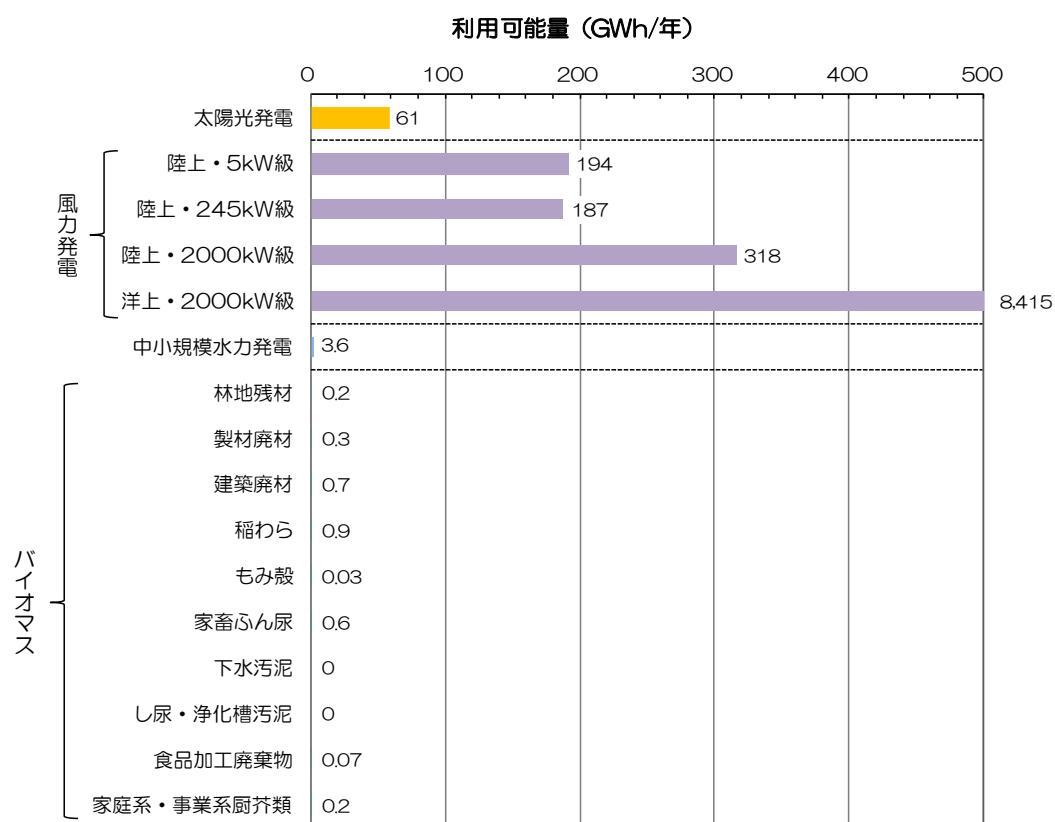
図4.3-1 エネルギー別 利用可能量（発電利用）
