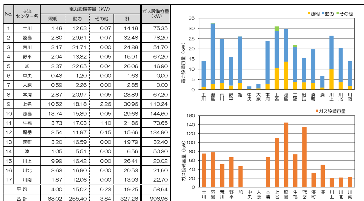
図4.6-2 交流センターの主要な設備容量（電力・ガス）
