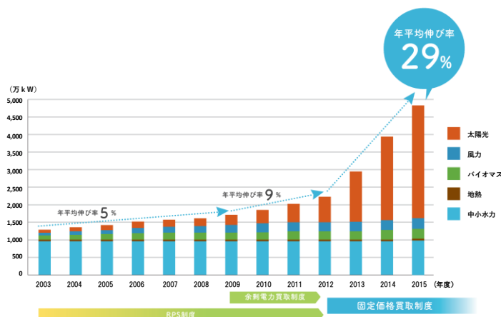
図4.2-1 全国における再生可能エネルギー等の設備容量の推移
