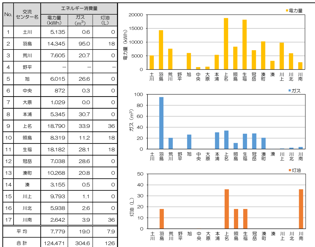
図4.6-3 交流センターの年間エネルギー消費量（電力量・ガス・灯油）
