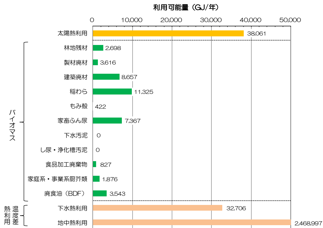
図4.3-3 エネルギー別 利用可能量（熱利用）
