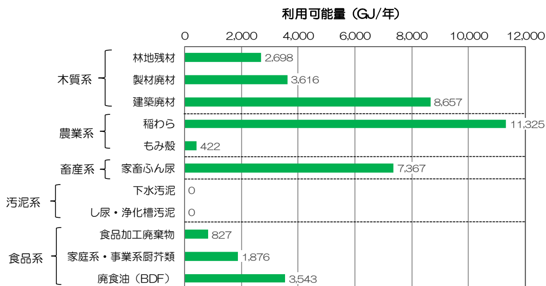
図4.3-4 バイオマス分類別 利用可能量（熱利用）
