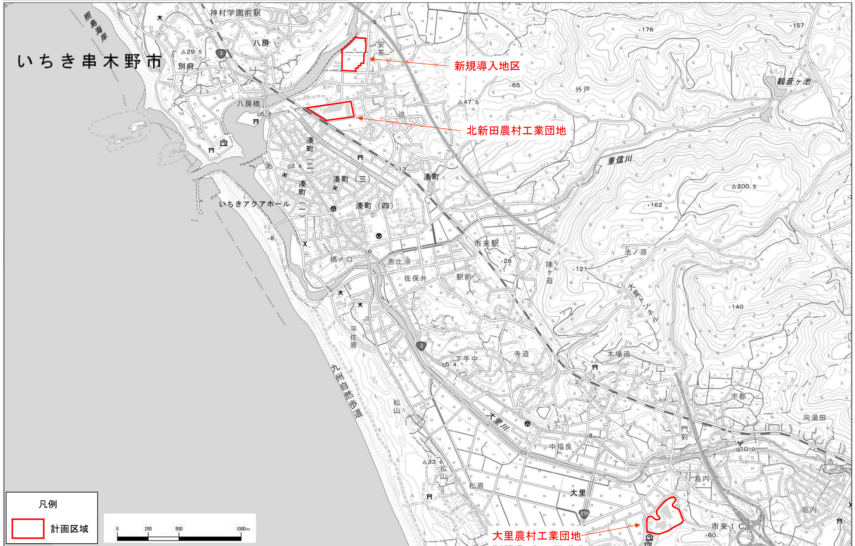
図 1 産業等導入地区位置図 S=1:15,000
