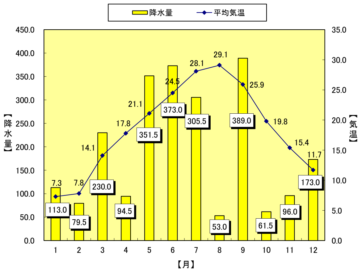
月別平均気温と降水量(平成30年)
