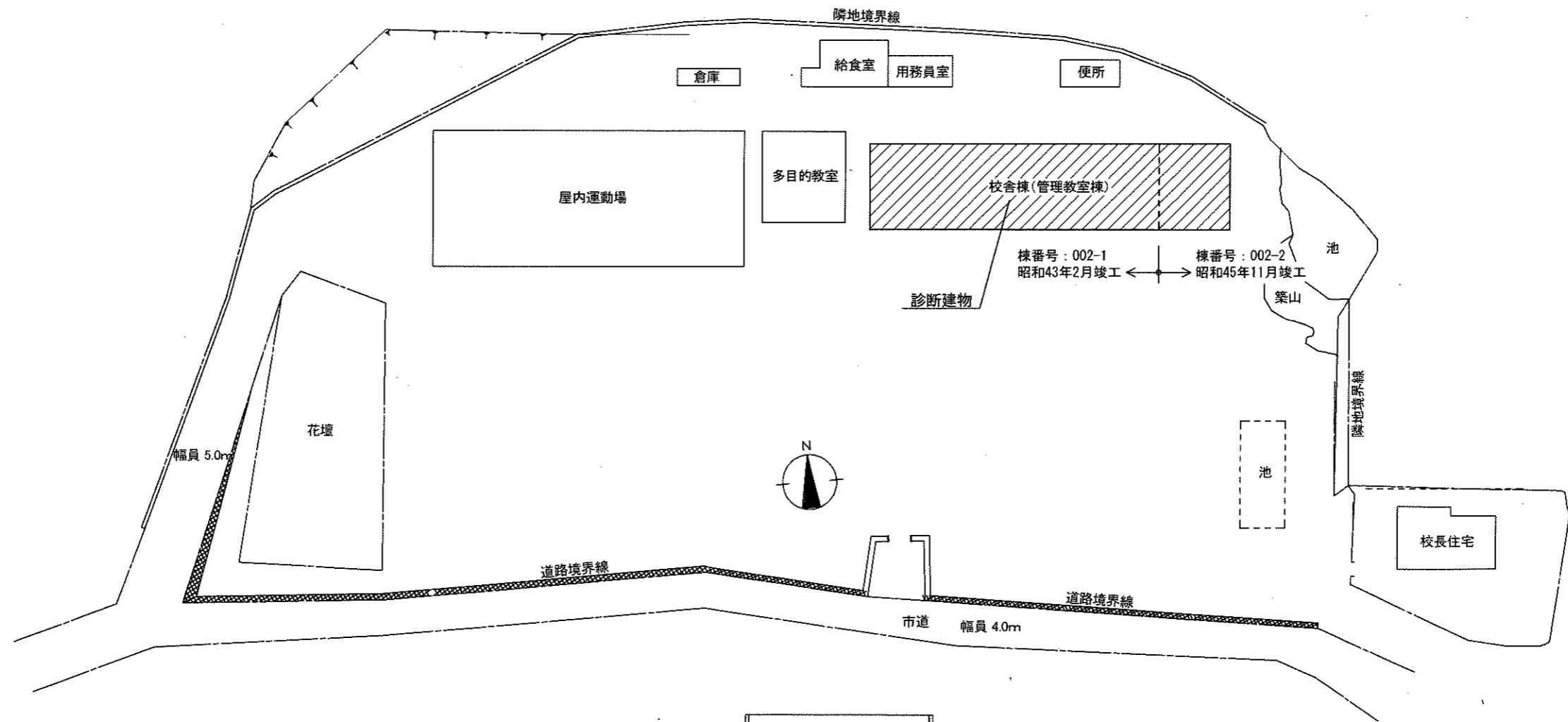
配置図 S=1/600
