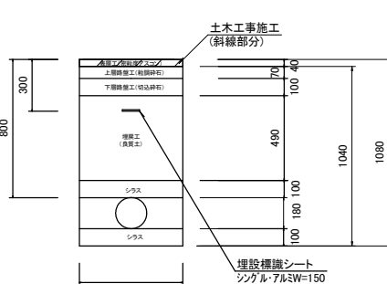
土工断面②(HPPEφ150) As舗装 H=800 S=1:20
