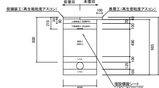
土工断面③(HPPEφ100) As舗装 H=800 S=1:20
