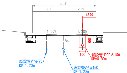
標準断面図 S=1:100
