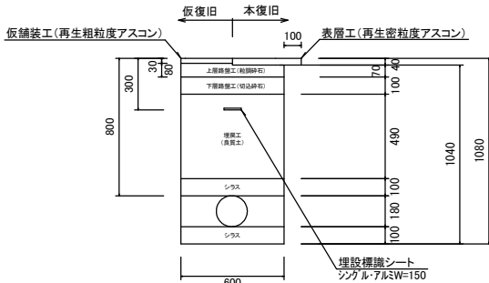
土工断面①(HPPEφ150) As舗装 H=800 S=1:20
