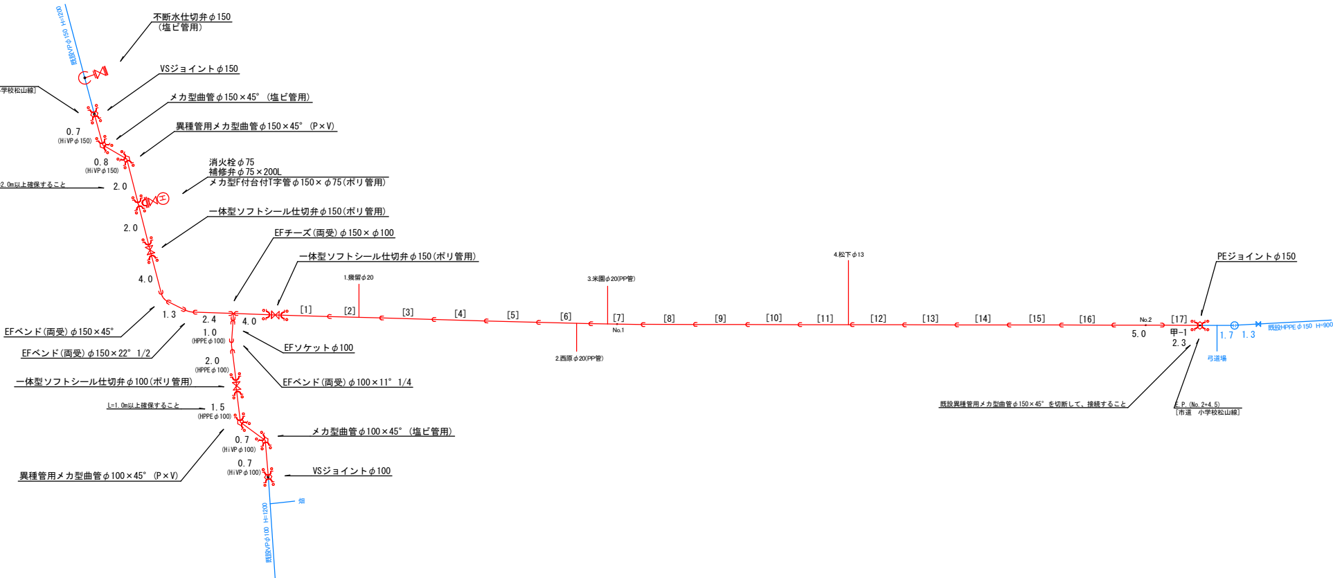
配管詳細図 S=1:250 [市道 小学校松山線]
