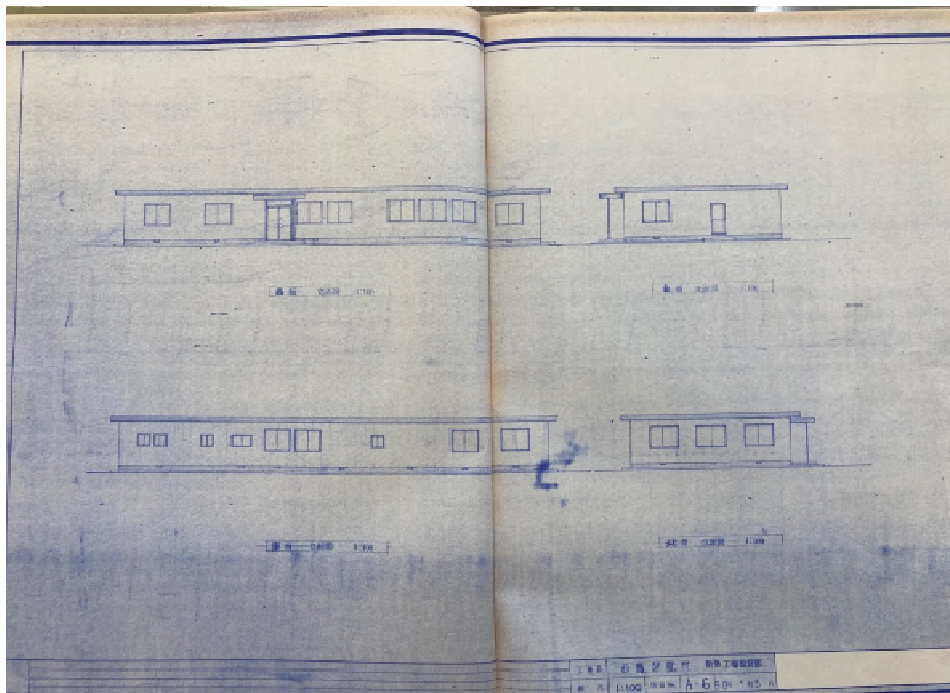
事務所棟図面
