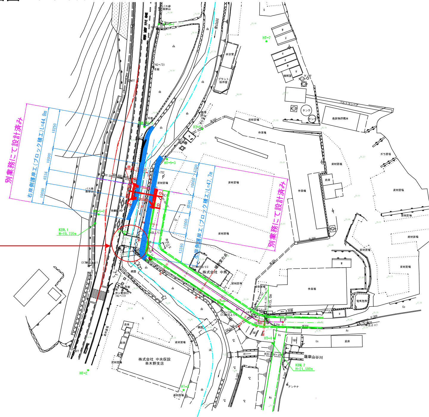
平面図 S=1:500
