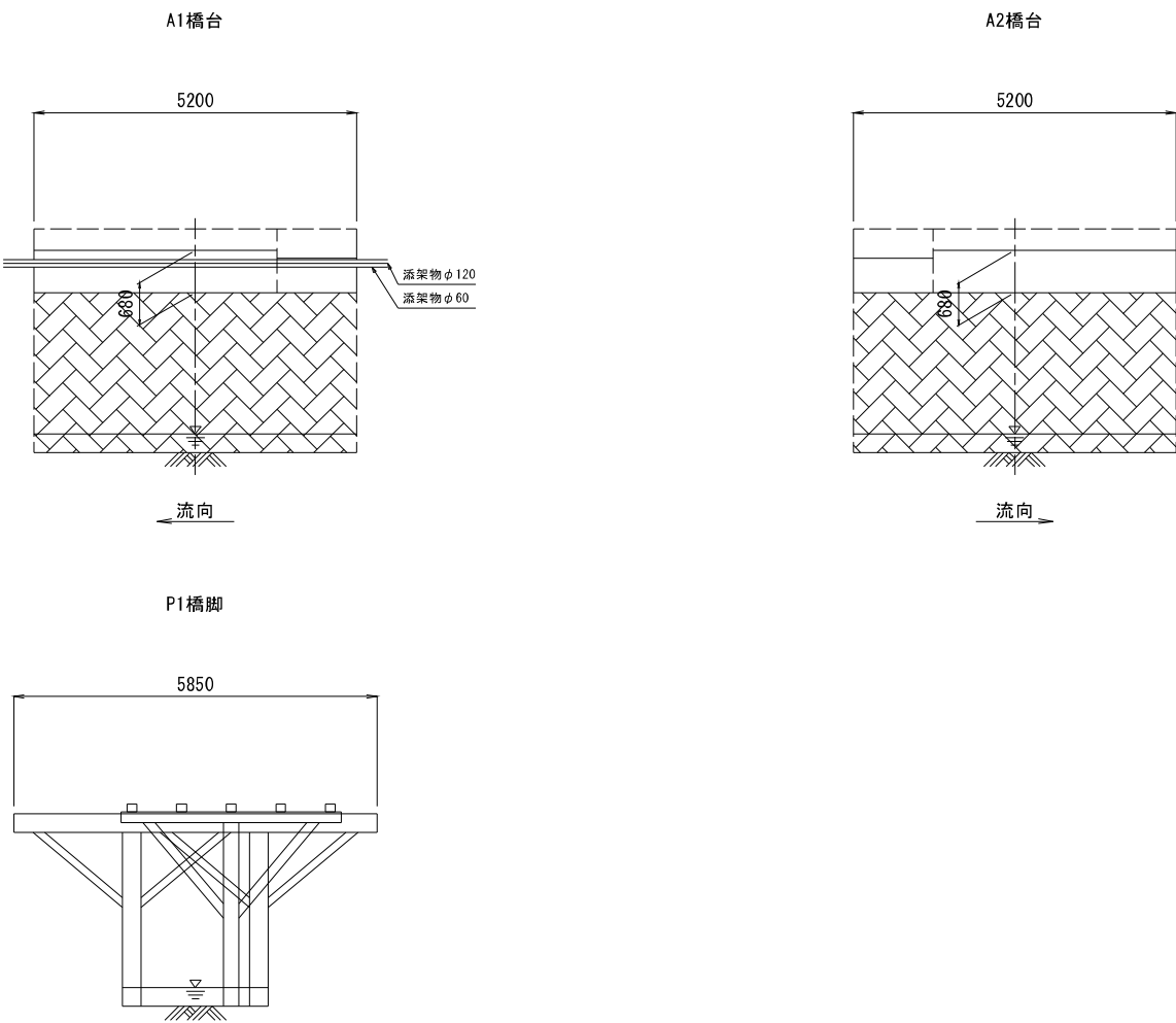
下部工正面図 S=1:60
