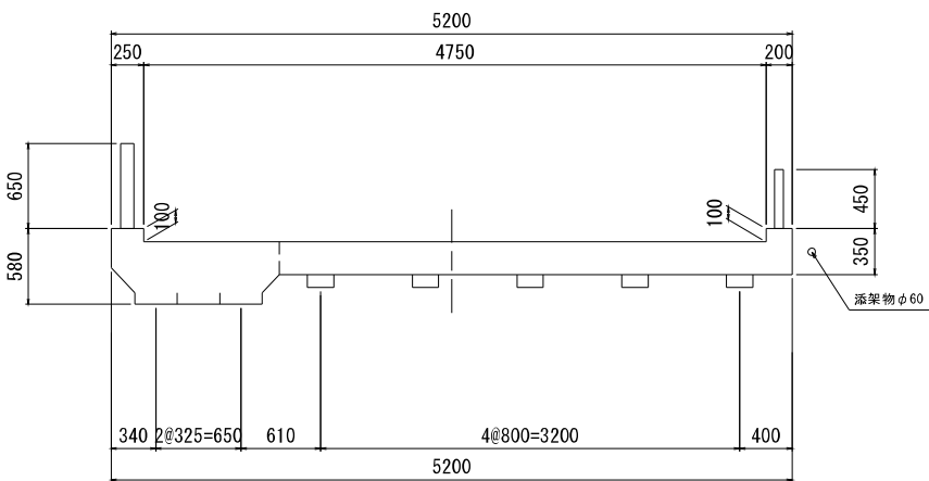
断面図 S=1:30
