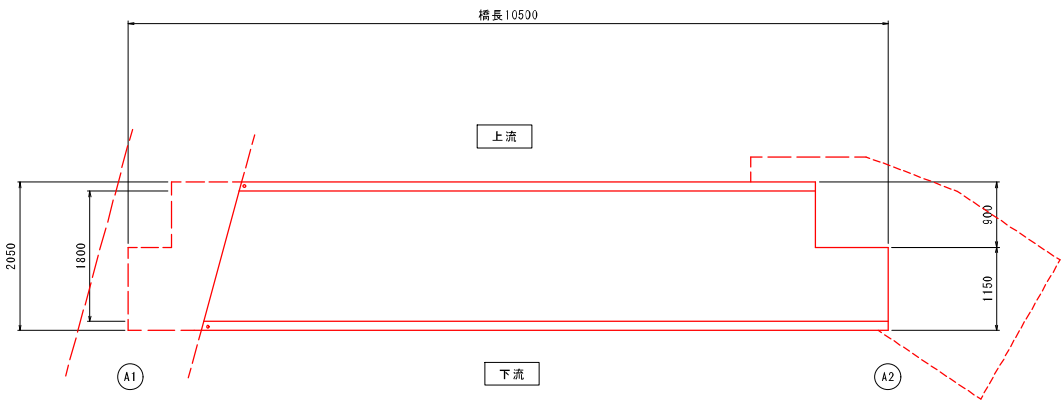
平面図 S=1:50
