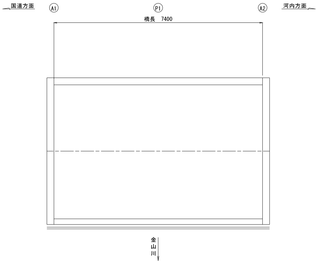
平面図 S=1:40
