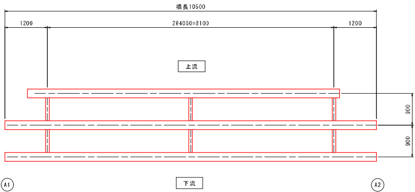
桁配置図 S=1:50
