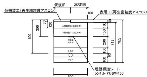
土工断面②(HPPE φ50) As舗装(車道)H=800 S=1:20
