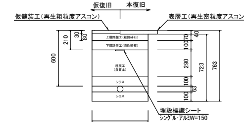
土工断面③(HPPE φ50) As舗装(車道)H=600 S=1:20
