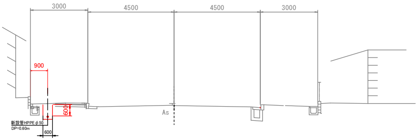
標準断面図 S=1:100
