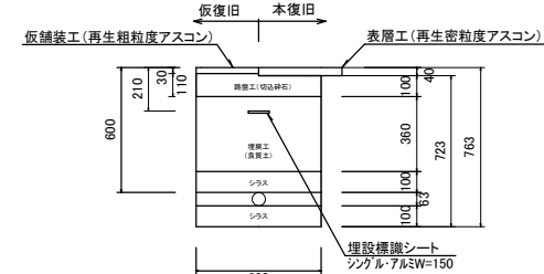
土工断面①(HPPE φ50) As舗装(歩道)H=600 S=1:20
